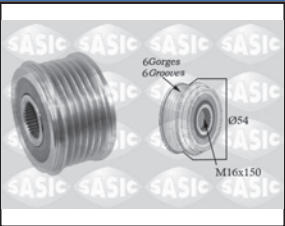
Ø ext. 54 M16x150
