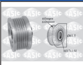
Ø ext. 61.5 M17x150
