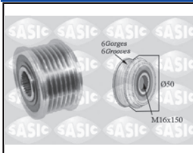
Ø ext. 50 M16x150
